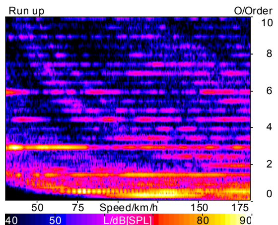
Figure 3 : Calcul sur la base du régime du moteur Représentation par rapport à la vitesse
