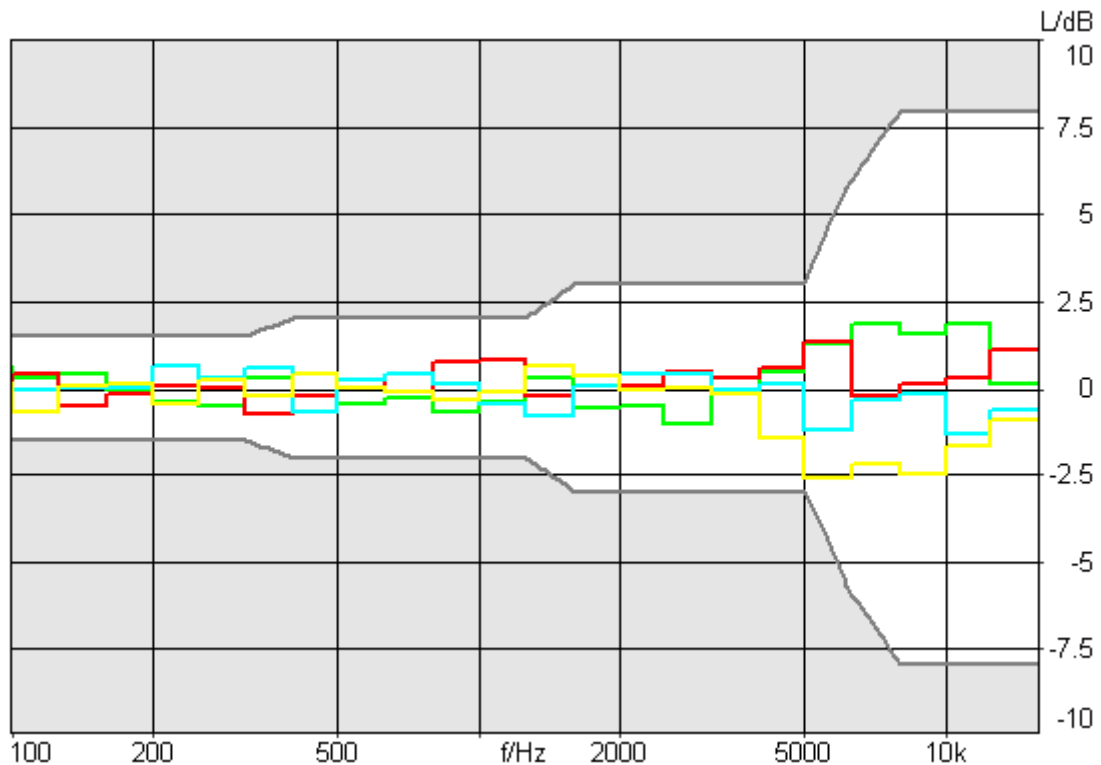
Abbildung 3.1: Vergleich von vier Messungen mit einem BHM, das von vier verschiedenen Personen getragen wurde (jede Kurve stellt jeweils die Differenz zum Mittelwert des rechten Kanals der Messung einer Person dar); zusätzlich sind die laut IEC 959 zulässigen Toleranzen für das Übertragungsverhalten eines Kunstkopfes im Freifeld als graue Kurven eingezeichnet
