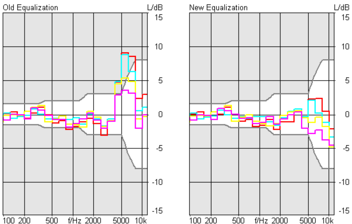
Abbildung 3.2: Unterschiede zwischen Kunstkopf- und BHM-Aufnahmen unter Verwendung der alten (linkes Diagramm) und neuen BHM-Entzerrung (rechtes Diagramm); zusätzlich sind die laut IEC 959 zulässigen Toleranzen für das Übertragungsverhalten eines Kunstkopfes im Freifeld als graue Kurven eingezeichnet
