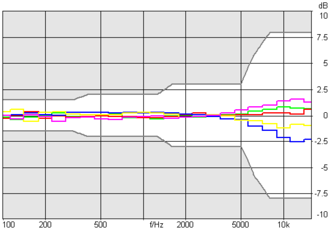
Abbildung 5.1: Vergleich des Übertragungsverhaltens von fünf verschiedenen BHS I (Differenz zum Mittelwert, jeweils der linke Kanal); zusätzlich sind die laut IEC 959 zulässigen Toleranzen für das Übertragungsverhalten eines Kunstkopfes im Freifeld als graue Kurven eingezeichnet
