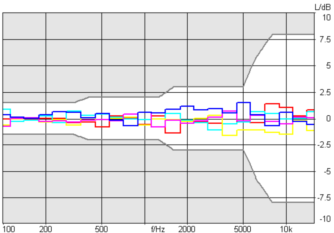
Abbildung 5.2: Vergleich des Übertragungsverhaltens eines BHS I, das von fünf verschiedenen Personen getragen wurde (Differenz zum Mittelwert, jeweils der linke Kanal); zusätzlich sind die laut IEC 959 zulässigen Toleranzen für das Übertragungsverhalten eines Kunstkopfes im Freifeld als graue Kurven eingezeichnet
