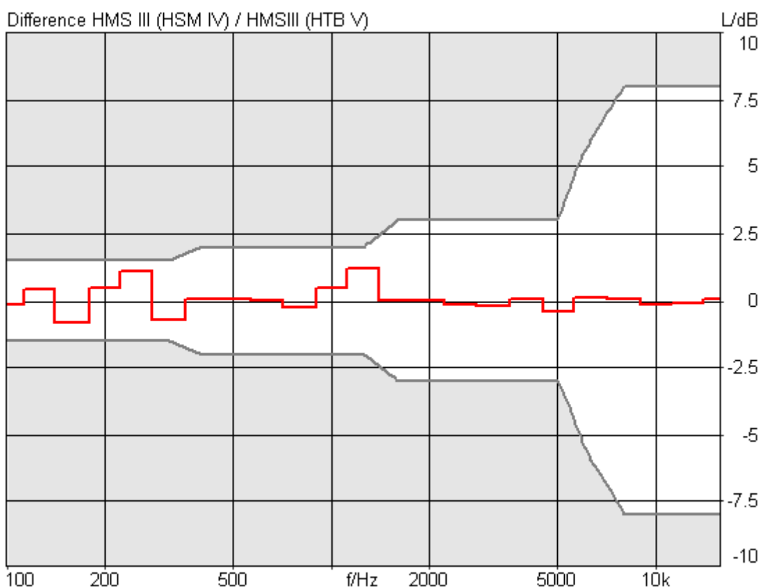
Abbildung 4.1: Vergleich zwischen einer Messung HMS III auf HSM IV und einer Messung HMS III auf HTB IV; zusätzlich sind die laut IEC 959 zulässigen Toleranzen für das Übertragungsverhalten eines Kunstkopfes im Freifeld als graue Kurven eingezeichnet
