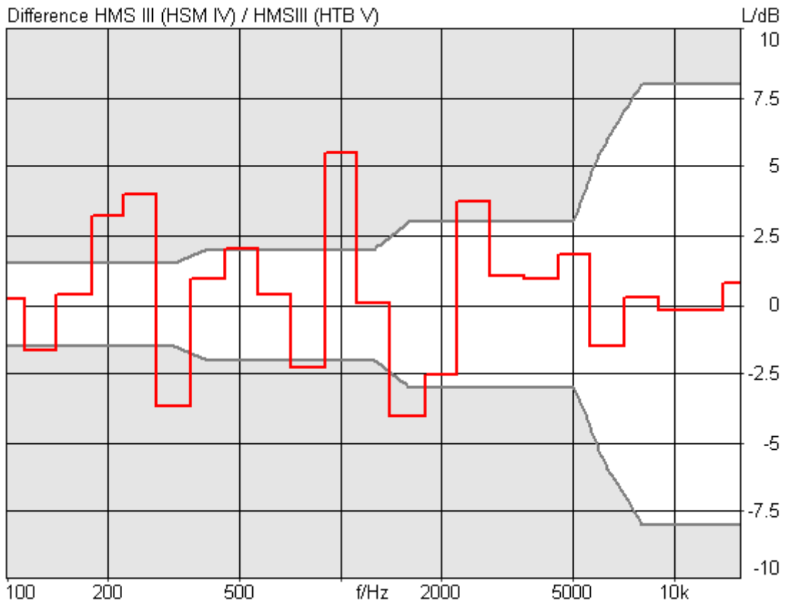
Abbildung 4.2: Vergleich zwischen einer Messung HMS III auf HSM IV und einer Messung HMS III auf HTB IV, ohne exakte Positionierung; zusätzlich sind die laut IEC 959 zulässigen Toleranzen für das Übertragungsverhalten eines Kunstkopfes im Freifeld als graue Kurven eingezeichnet
