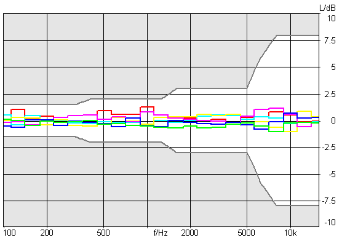
Abbildung 1.1: Vergleich des Übertragungsverhaltens von sechs verschiedenen Kunstköpfen (Differenz zum Mittelwert, jeweils der linke Kunstkopfkanal); zusätzlich sind die laut IEC 959 zulässigen Toleranzen für das Übertragungsverhalten im Freifeld als graue Kurven eingezeichnet
