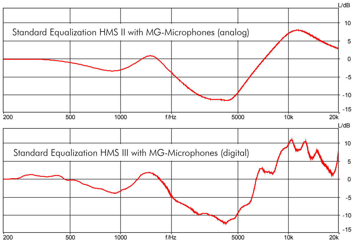
Abbildung 2.1: Vergleich einer HMS-II-Entzerrung (analog) mit einer HMS-III-Entzerrung (digital)
